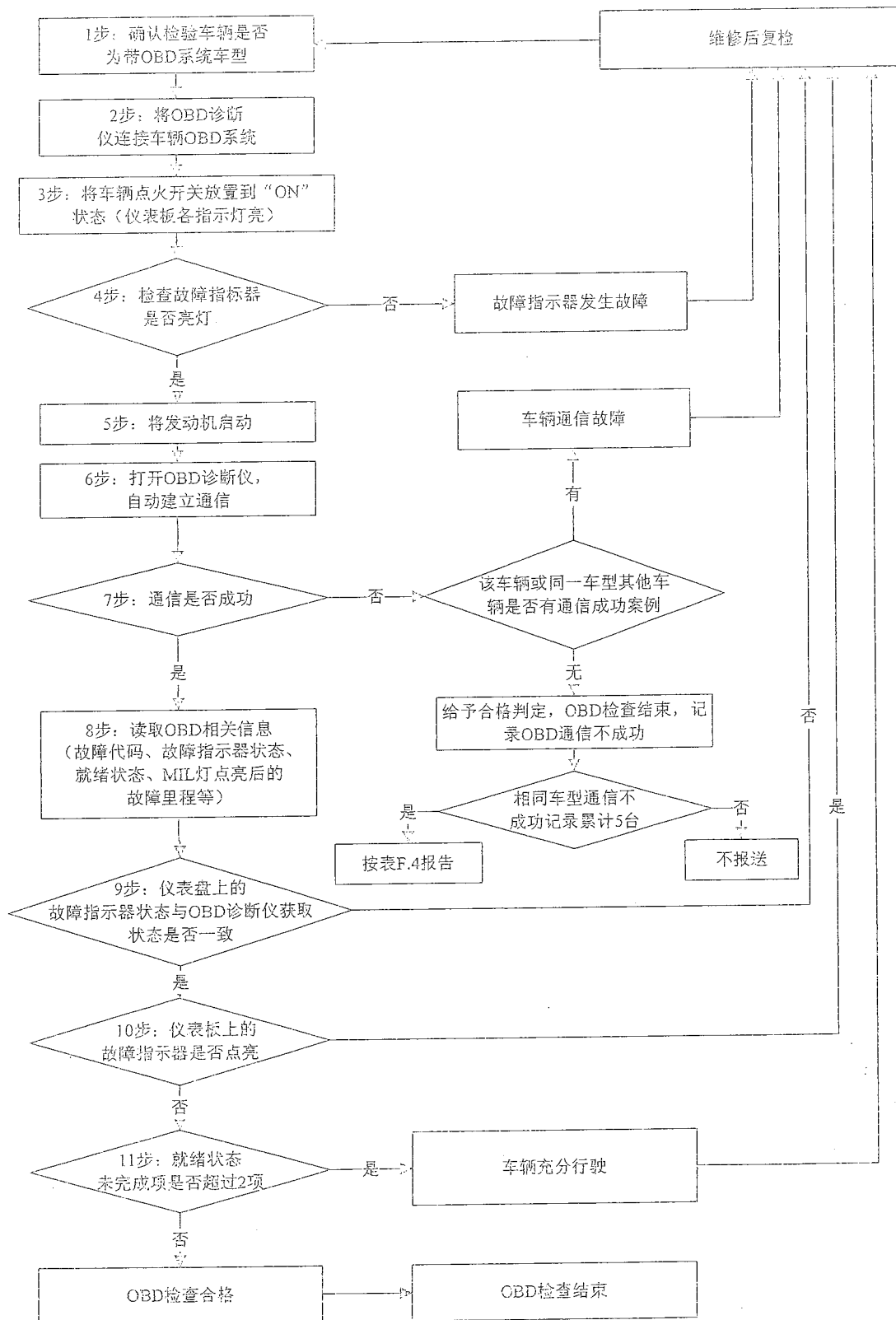
图 E.1 OBD 系统检查流程示意图
